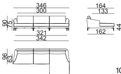
CHAISE LONGUE 346
