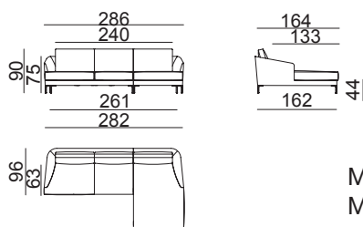
CHAISE LONGUE 346
