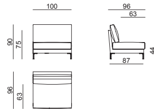
MOD. 100
