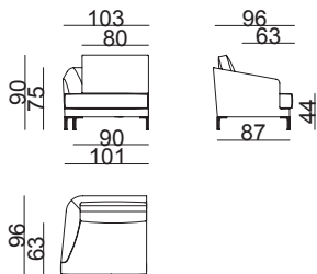
MOD. 90
