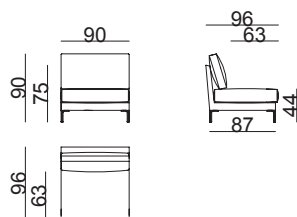
MOD. 90
